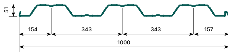
TẤM SÀN | DECKING PANEL
