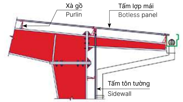
MÁI VƯỢN TƯỜNG BIÊN SIDEWALL ROOF EXTENTION
