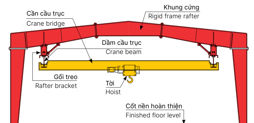
CẦU TRỤC CHẠY DƯỚI | UNDERHUNG CRANES
