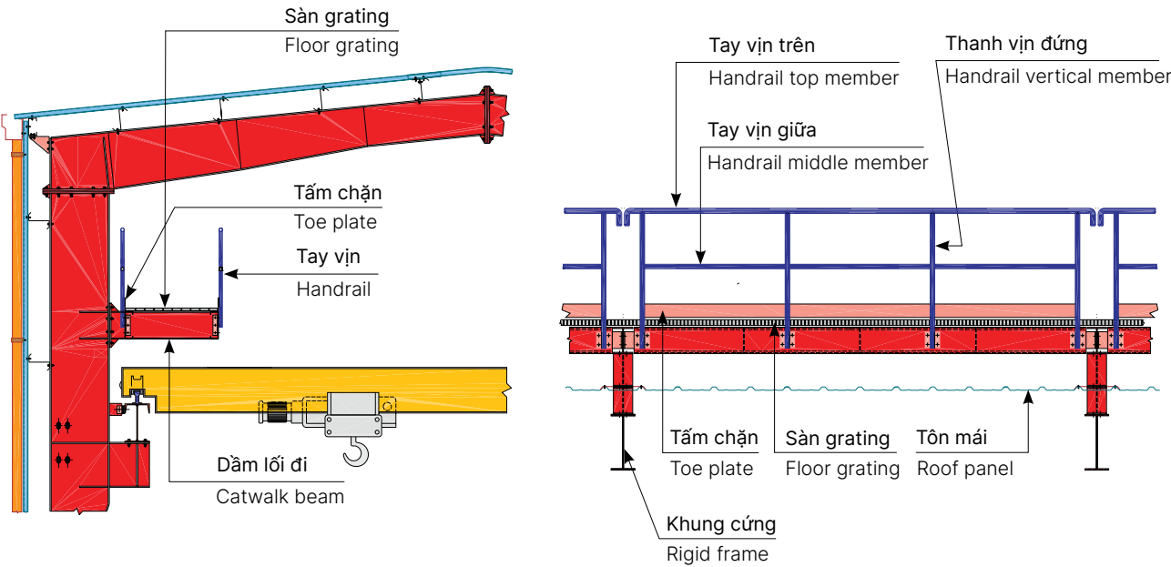
LỐI ĐI TRÊN CỘT KHUNG CỨNG CATWALKS AT RIGID FRAME COMLUNM
