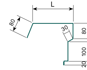
DIỀM MÁI ĐẦU HỒI | GABLE TRIM
