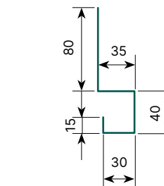
DIỀM CHÂN TÔN | DRIP TRIM
