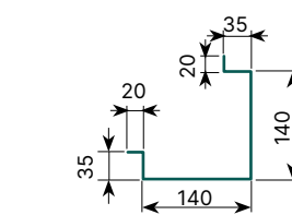
DIỀM CHỐNG TẠT CHÂN NÓC GIÓ FLASHING FOR ROOF MONITOR
