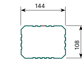
ỐNG XỐI TÔN | DOWNSPOUT
