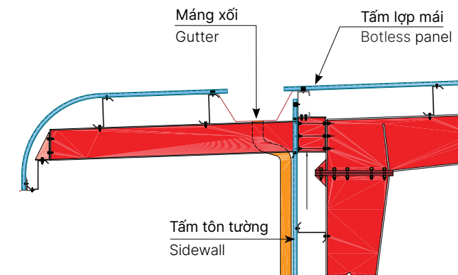
MÁI ĐUOA CONG CURVED CANOPY
