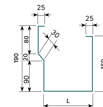
MÁNG XỐI BIÊN | EAVE GUTTER
