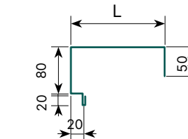
DIỀM ĐỈNH | CAP FLASHING
