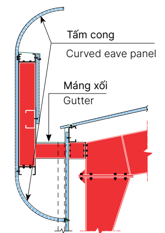
MẶT DỰNG CONG TRÊN DƯỚI TOP & BOTTOM CURVED FASCIA
