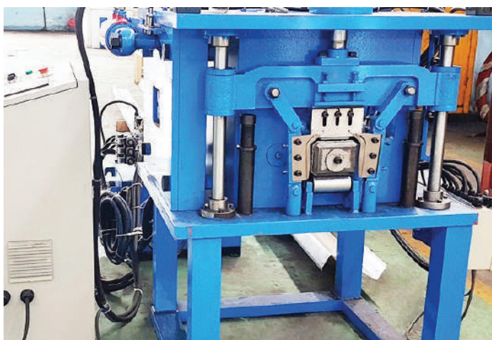
5.10 MÁY CÁN CO ỐNG XÓI THOÁT NƯỚC
