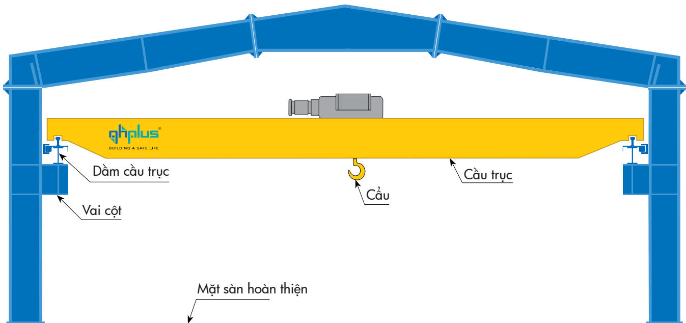
KHUNG KÈO CÓ CẦU TRỤC DI ĐỘNG (TPR-CRN)
