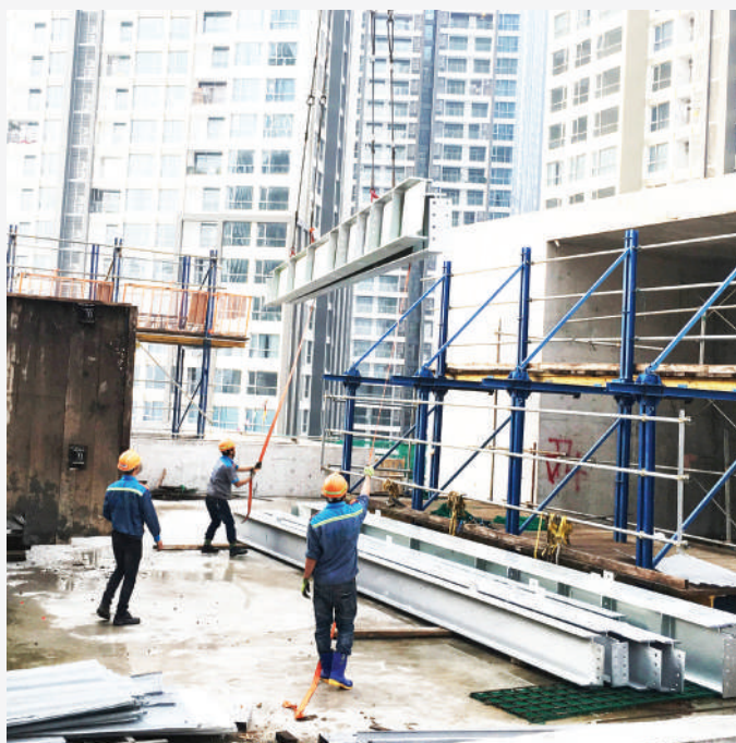
LẮP DỰNG KẾT CẤU LÒI THÉP CÔNG TRÌNH TÒA CAO ỐC LANDMARK 81
