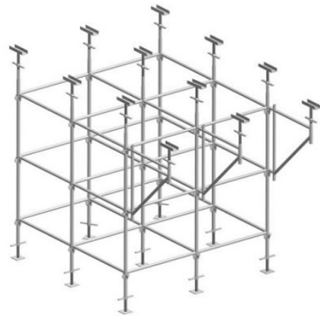
GIÀN GIÁO NÊM 楔形脚手架
