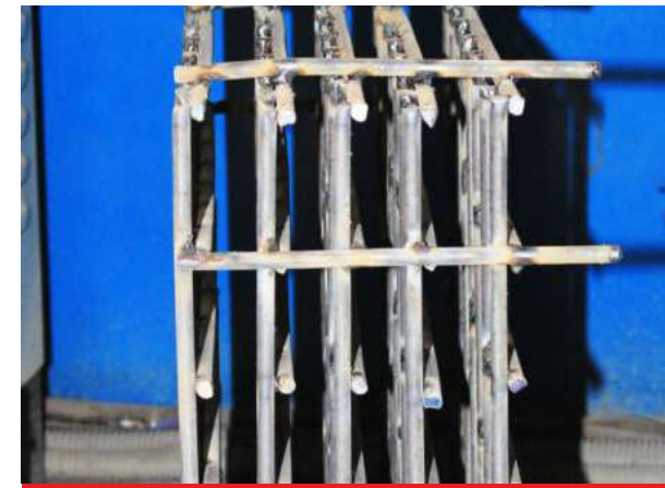
LƯỚI CỐT THÉP DỌC
