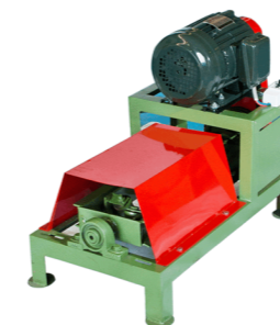
MÁY DUỖI SẮT DSM114 1HP 220V DSM114 IRON STRETCHING MACHINE 1HP 220V
